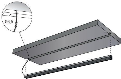
6010001 Clip di fissaggio (incluso) Fixing clip (included) Befestigungsclip (inbegriffen)
